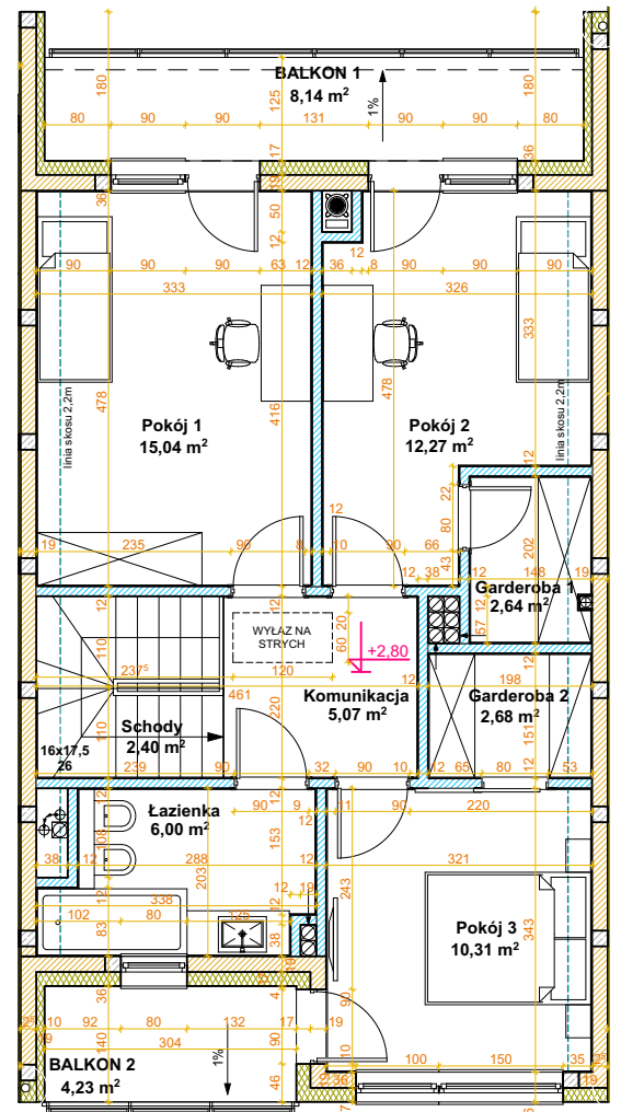
RZUT PODDASZA
