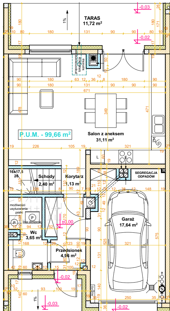
RZUT PARTERU
