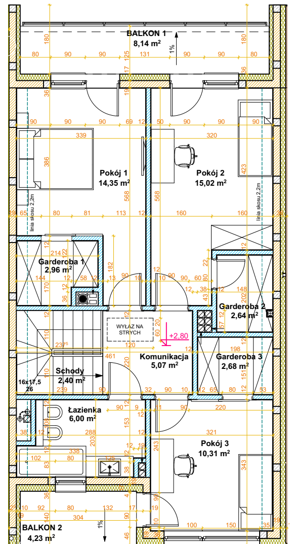
RZUT PODDASZA
