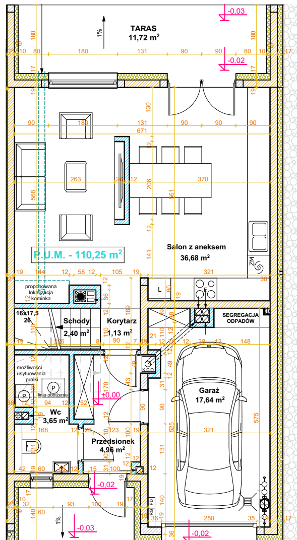
RZUT PARTERU
