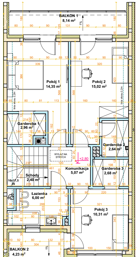
RZUT PODDASZA
