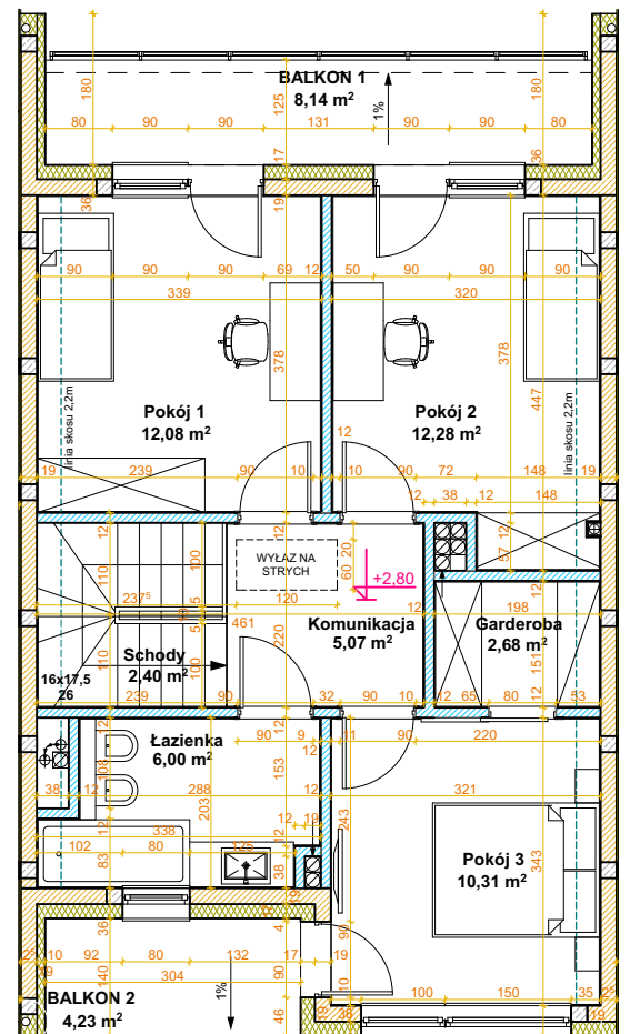
RZUT PODDASZA
