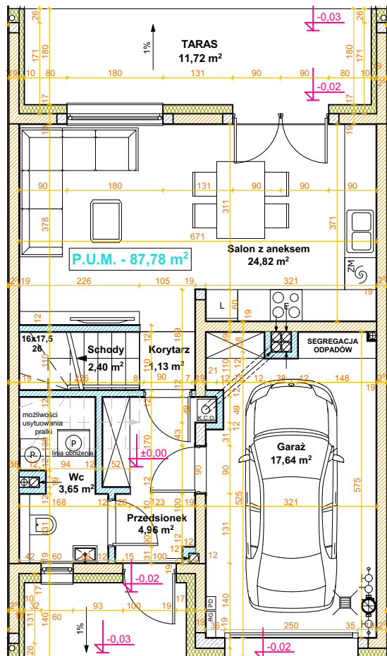
RZUT PARTERU
