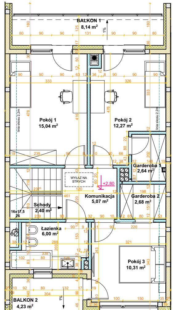
RZUT PODDASZA
