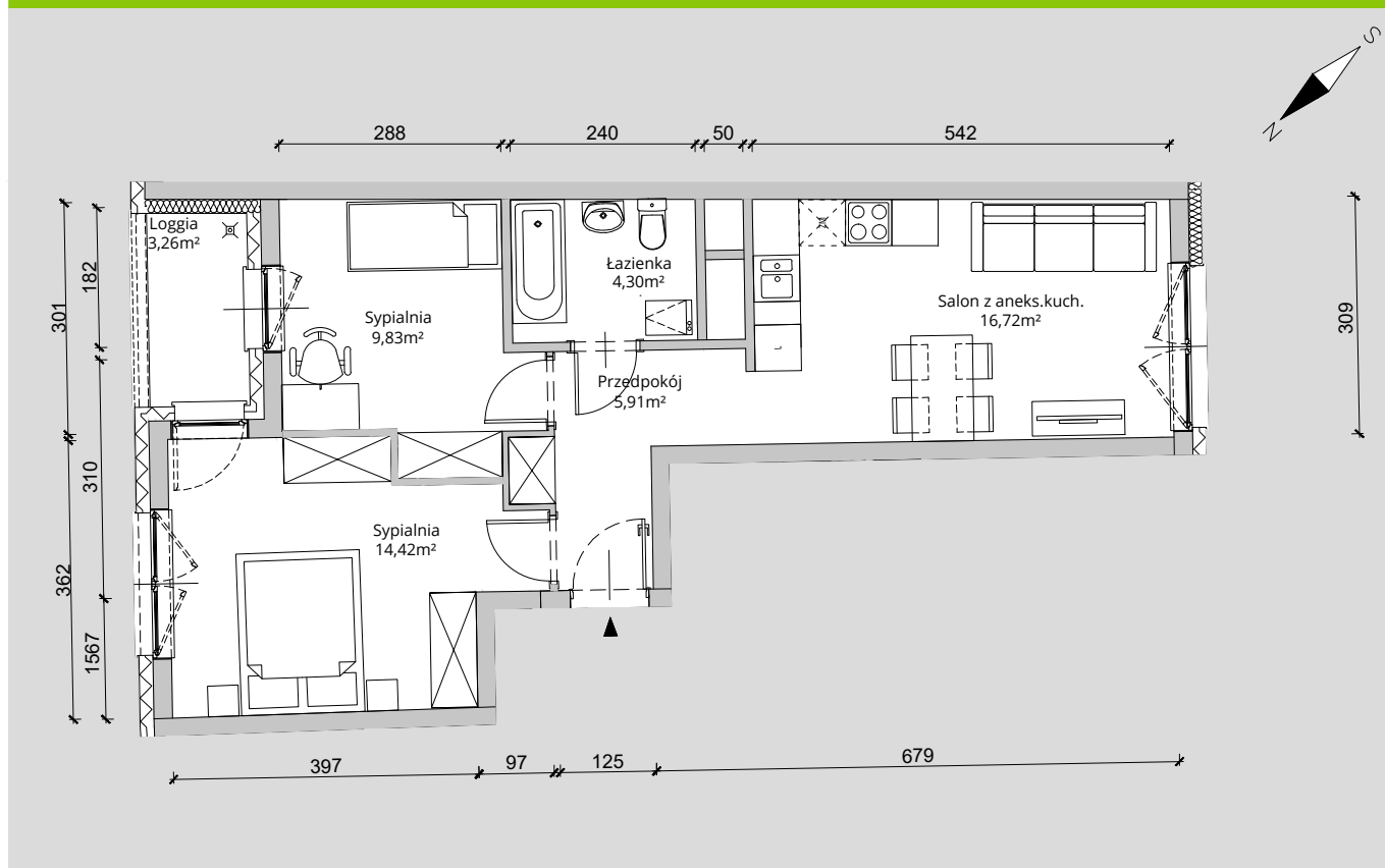
RZUT KONDYGNACJI 3 PIĘTRO
