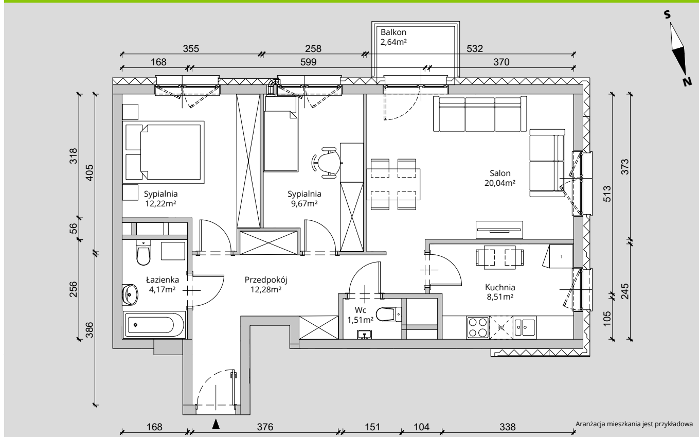
RZUT KONDYGNACJI 5 PIĘTRO
