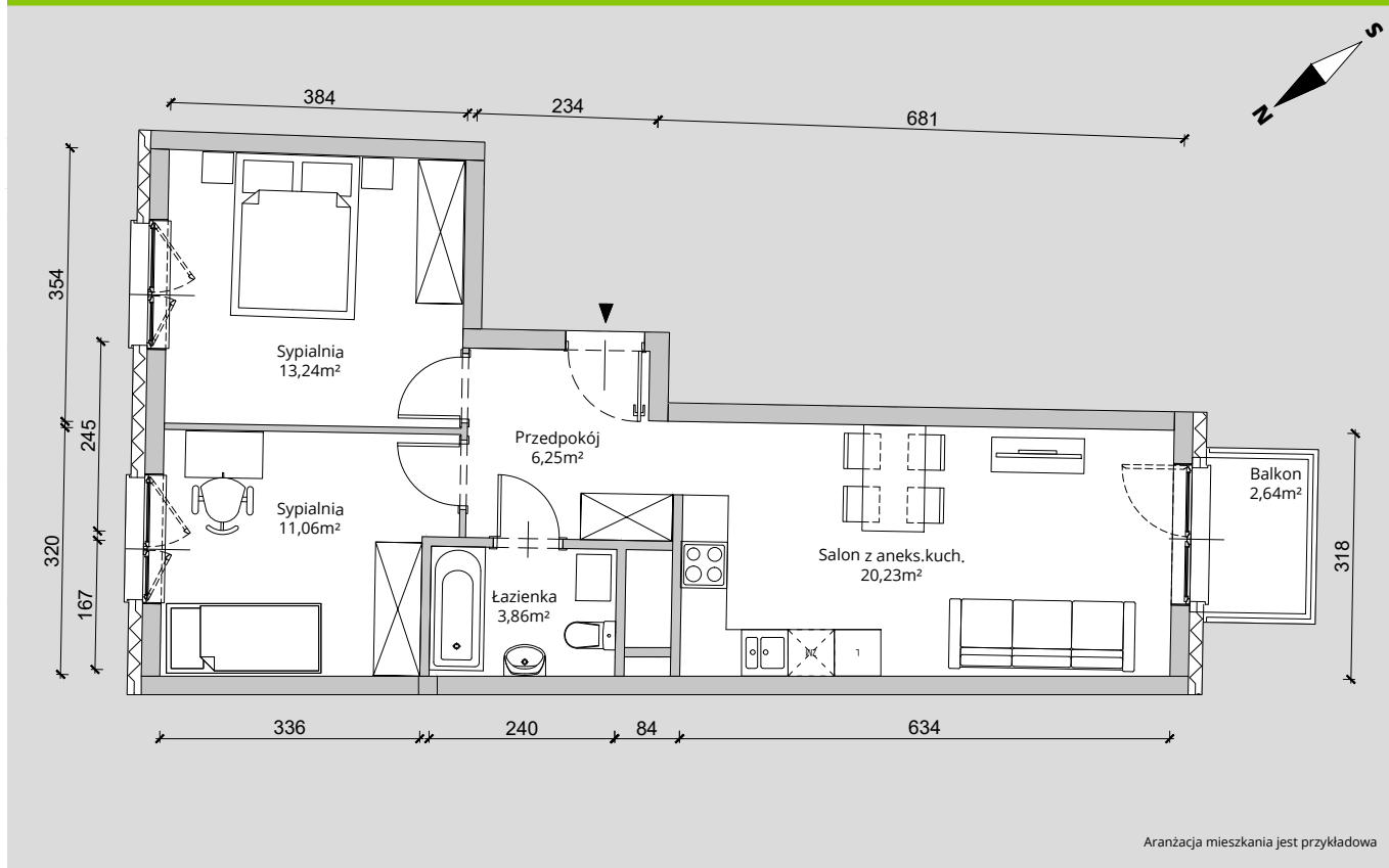
RZUT KONDYGNACJI 6 PIĘTRO
