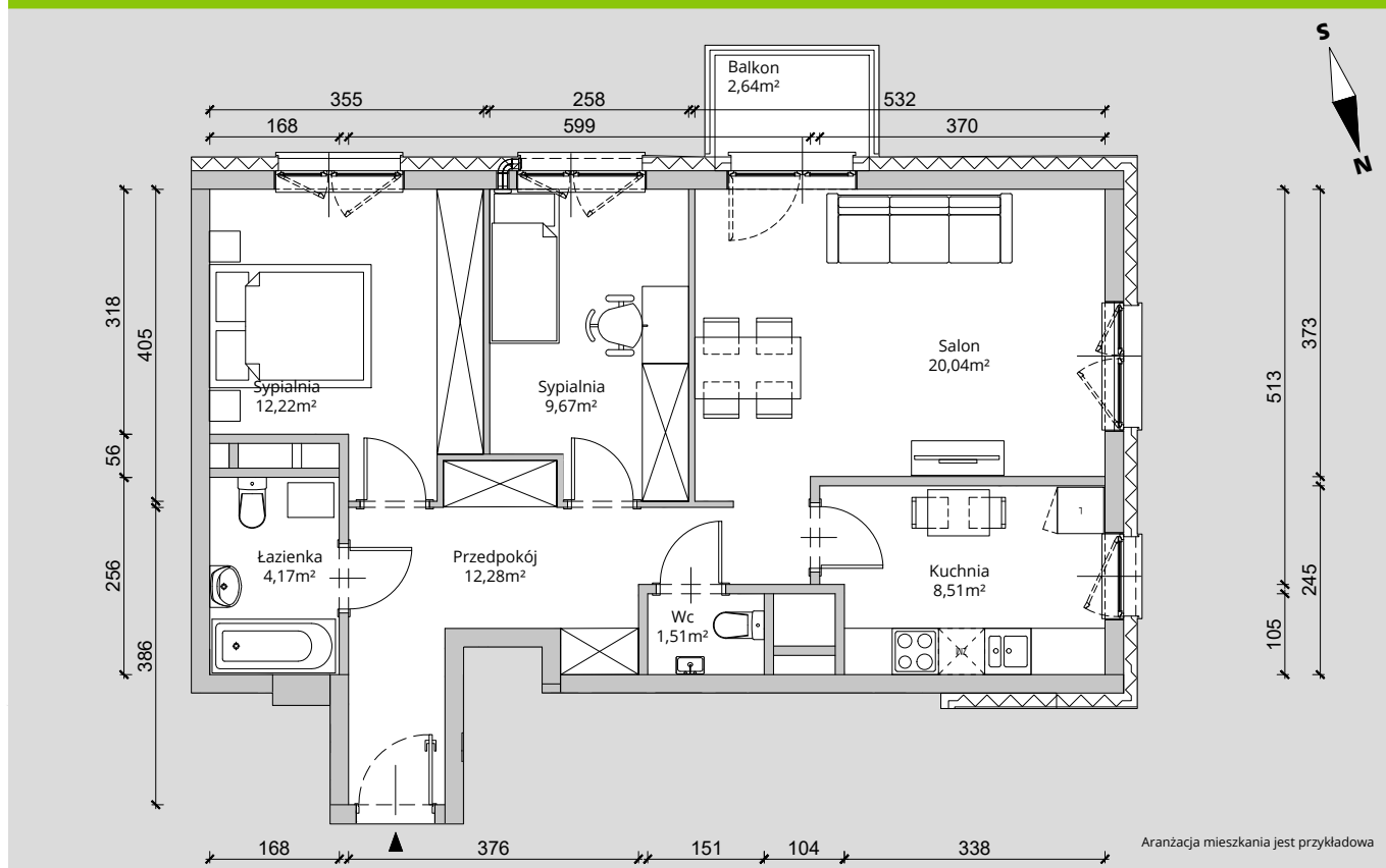
RZUT KONDYGNACJI 4 PIĘTRO
