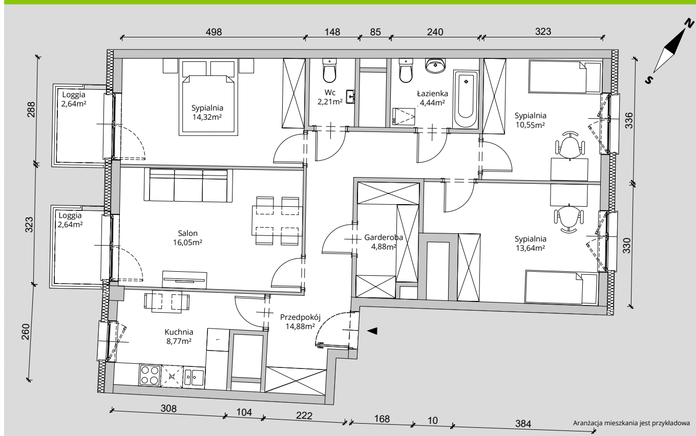
RZUT KONDYGNACJI 11 PIĘTRO
