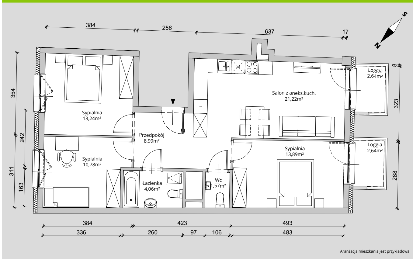
RZUT KONDYGNACJI 10 PIĘTRO
