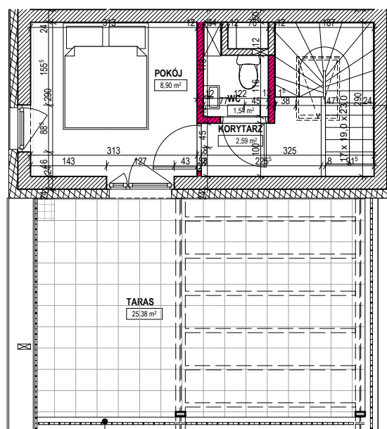
POZIOM PODDASZA UŻYTKOWEGO
