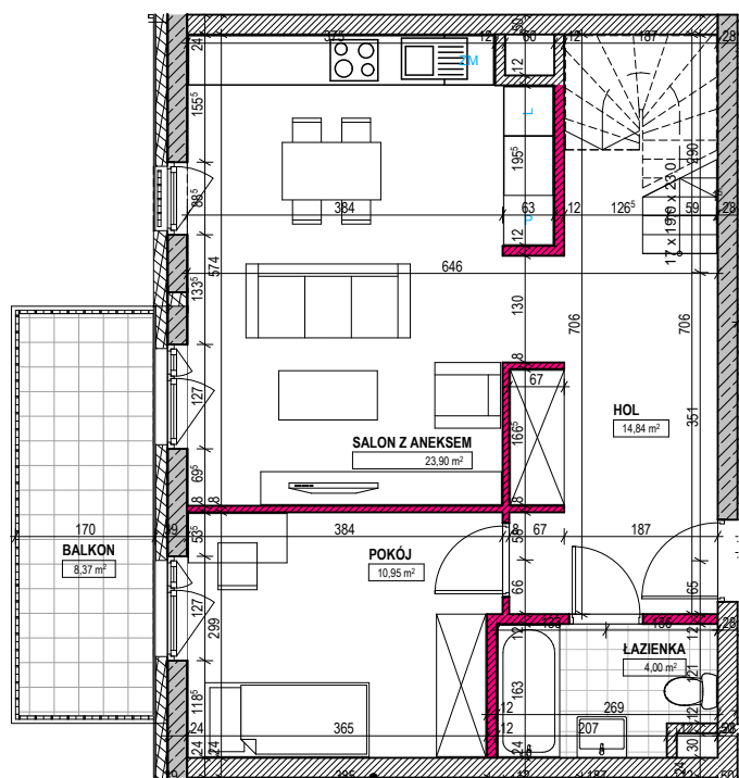
POZIOM TRZECIEGO PIĘTRA
