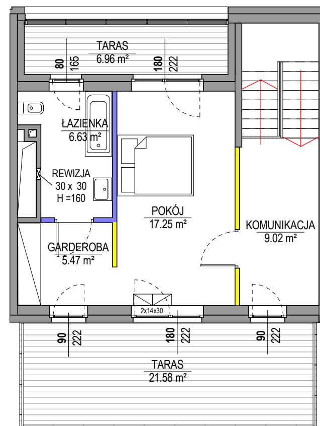
2. PIĘTRO
