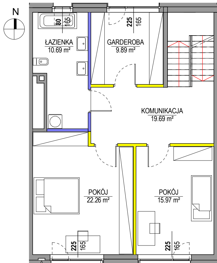
1. PIĘTRO
