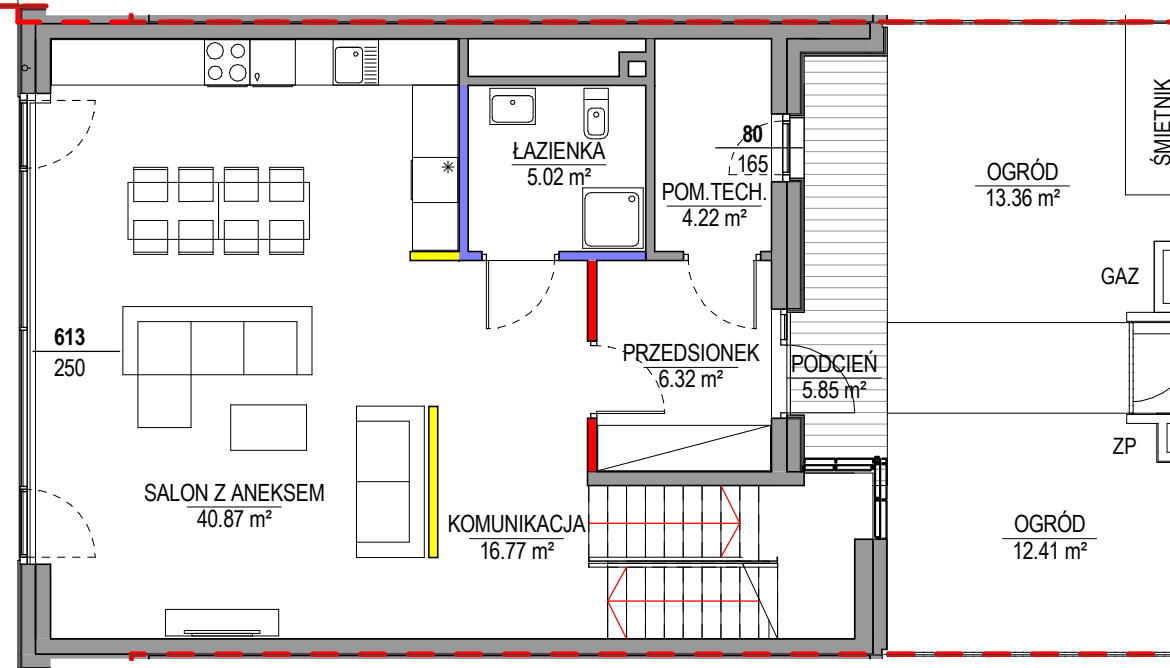
KONDYGNACJA -1
