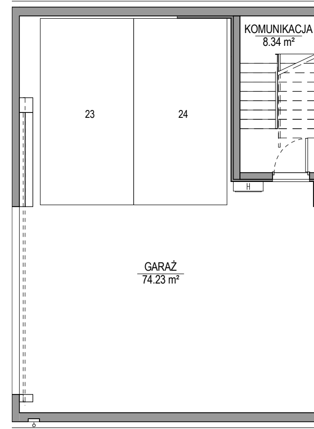
KONDYGNACJA -1
