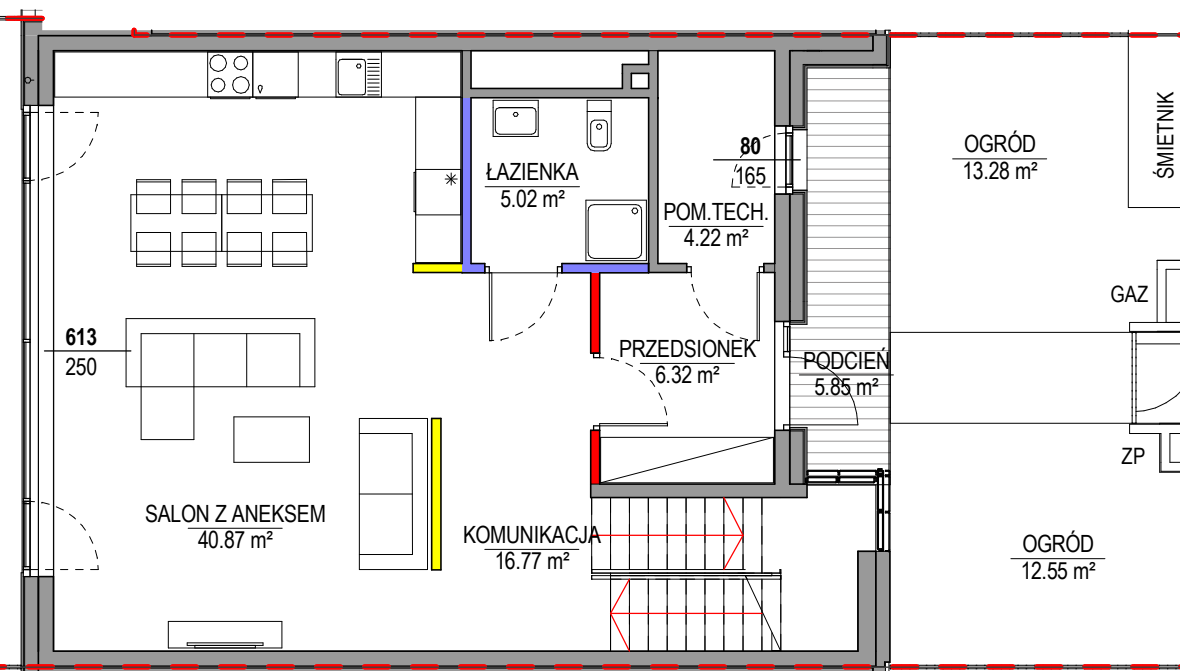
KONDYGNACJA -1
