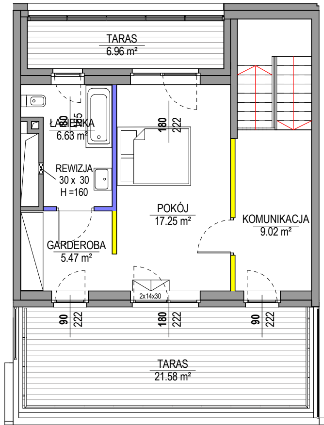
2. PIĘTRO
