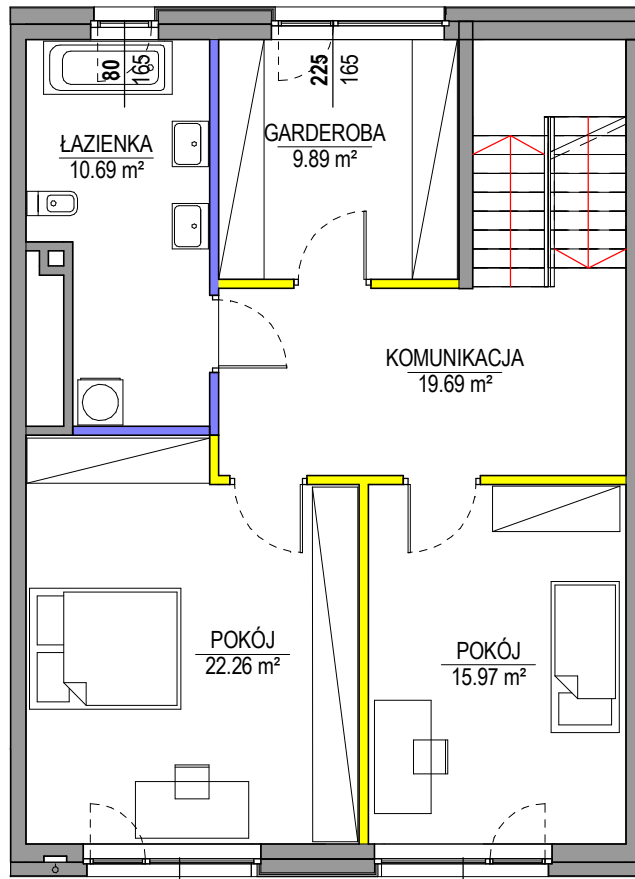
1. PIĘTRO
