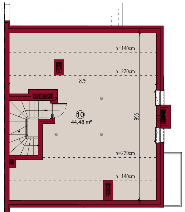
RZUT PODDASZA NIEUŻYTKOWEGO
