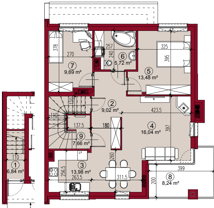
RZUT PARTERU
