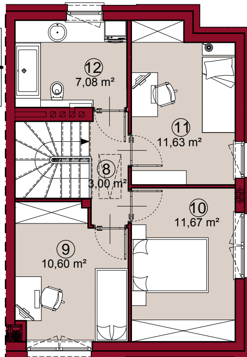
RZUT PIĘTRA
