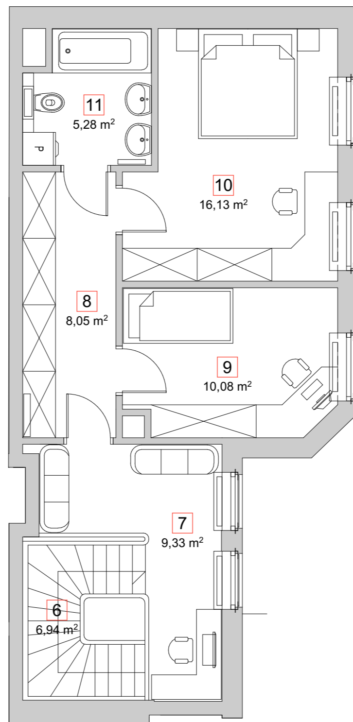
RZUT V PIĘTRA
