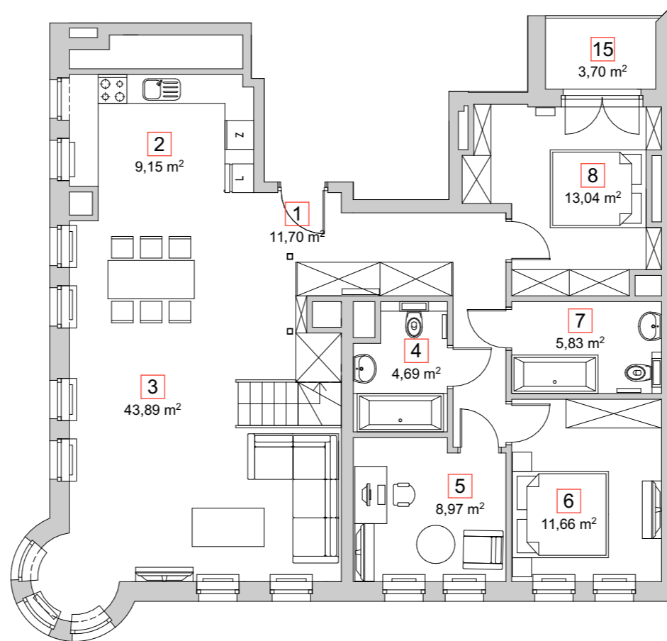
RZUT V PIĘTRA
