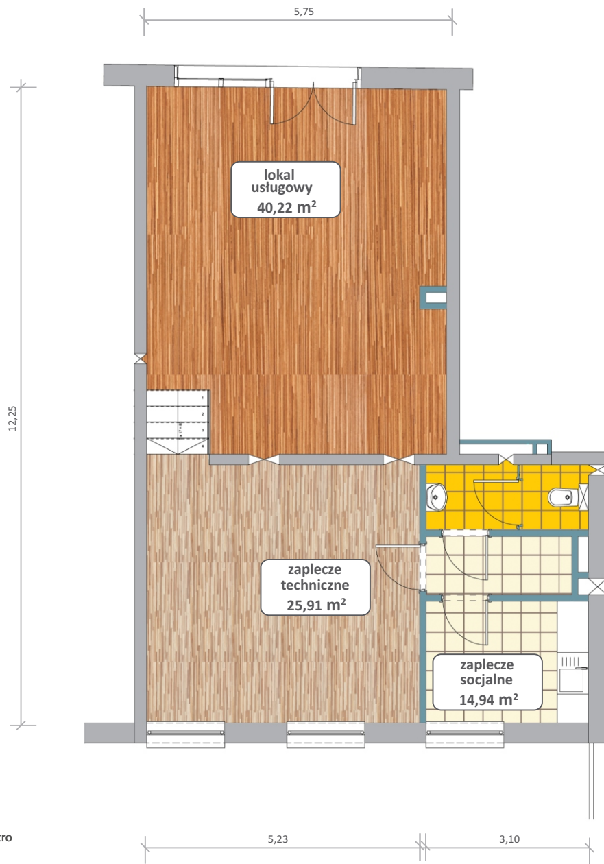
Rzut lokalu
