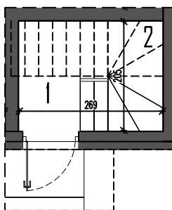
RZUT PARTERU
