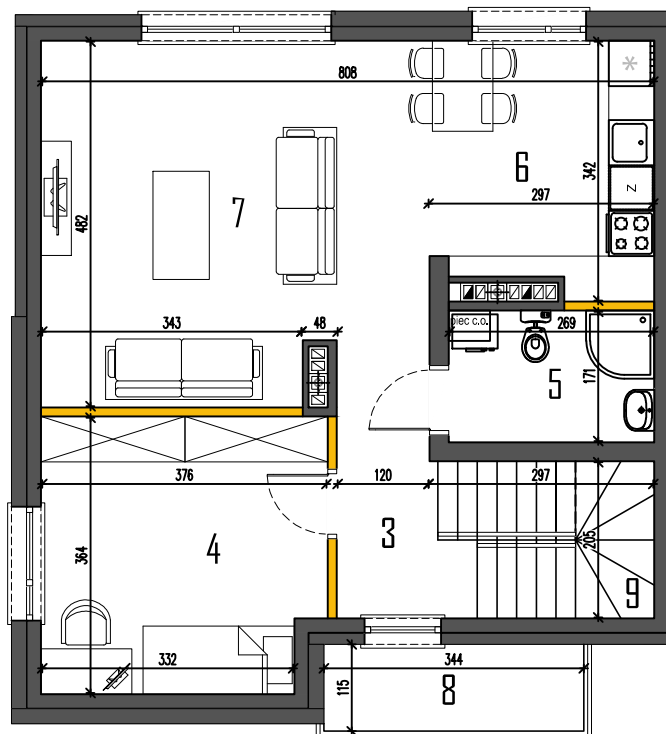
RZUT PIĘTRA
