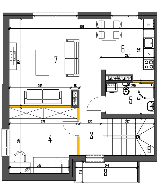
RZUT PIĘTRA
