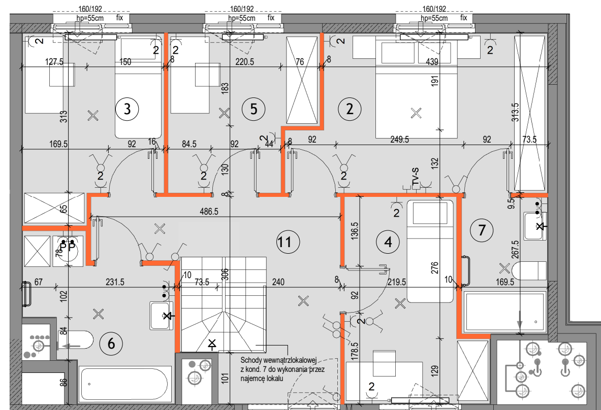
POZIOM GÓRNY
