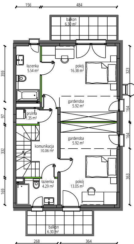
I PIĘTRO
