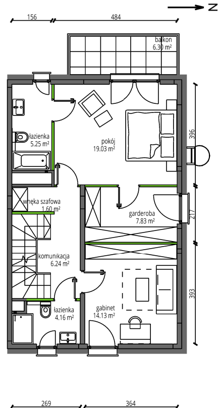
II PIĘTRO
