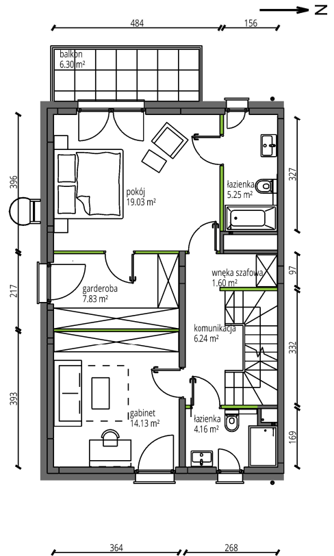
II PIĘTRO
