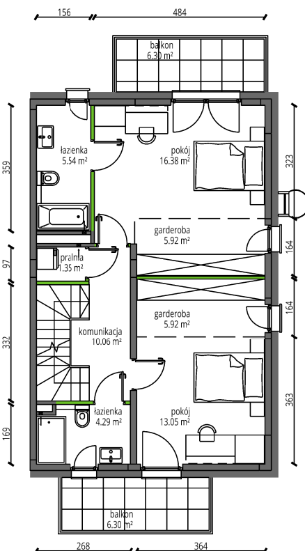
I PIĘTRO
