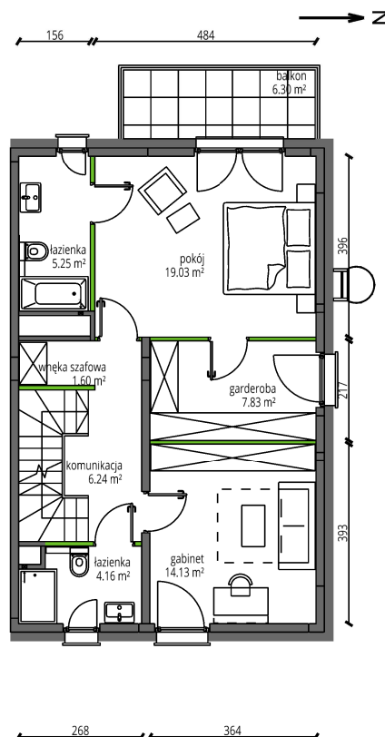
II PIĘTRO
