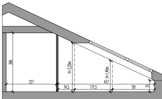
PRZESZKÓJ A-A
