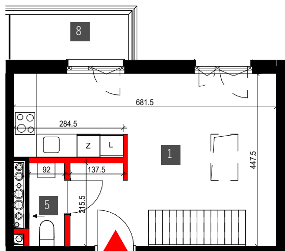
kondygnacja +3
