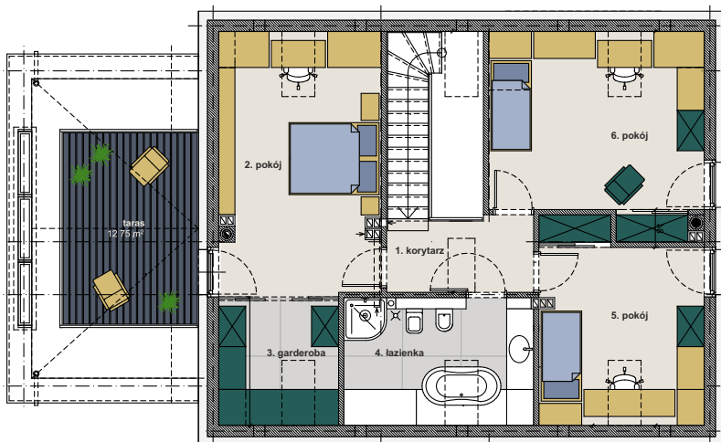
Rzut poddasza
