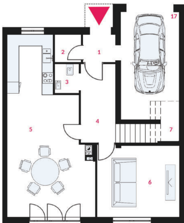
RZUT PARTERU
