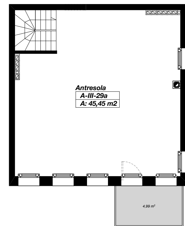
Rzut antresoli skala 1:100
