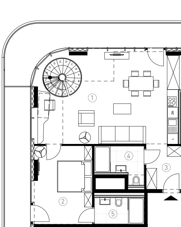
poziom 1 (71,56m 2 )
