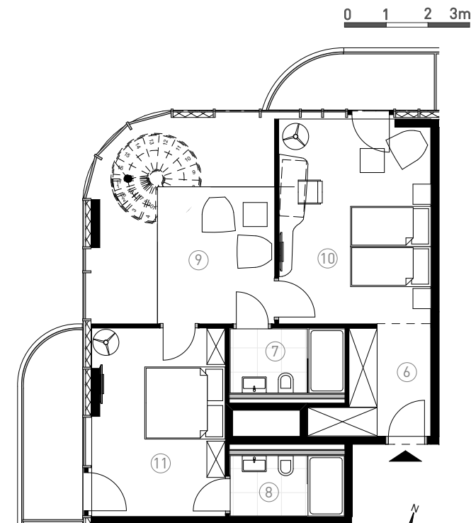
poziom 2 (59,49m 2 )
