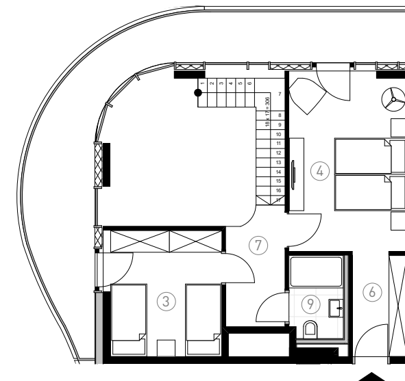
poziom 2 (39,75m 2 )
