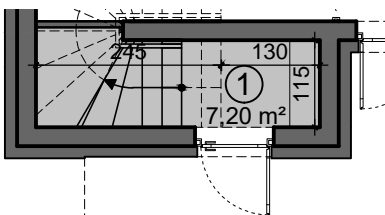
RZUT PARTERU
