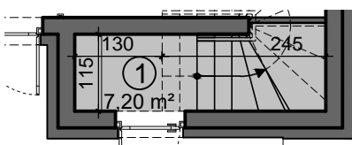
RZUT PARTERU
