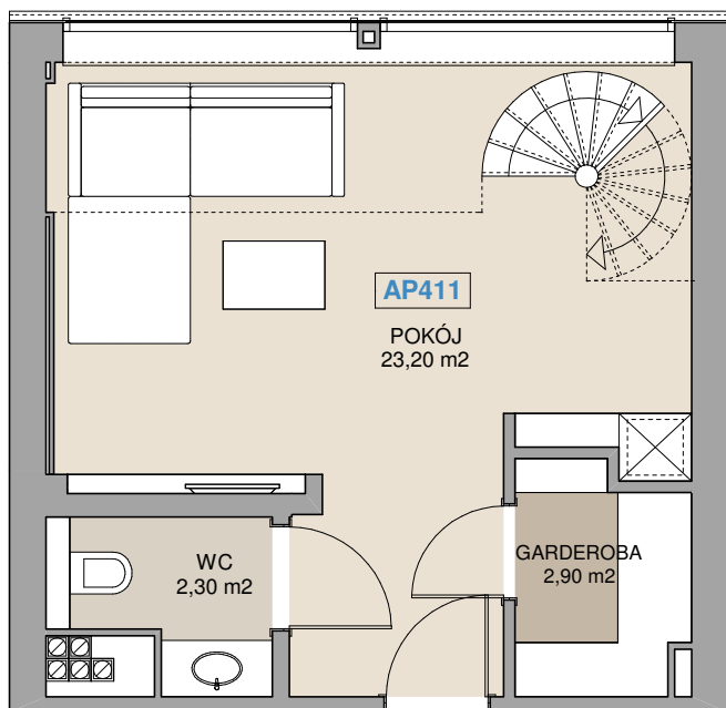
POZIOM 0- 28,40m 2
