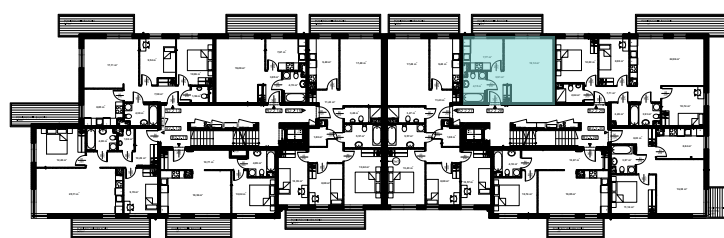
Klatka A Klatka B Rzut kondygnacji - II piętro
