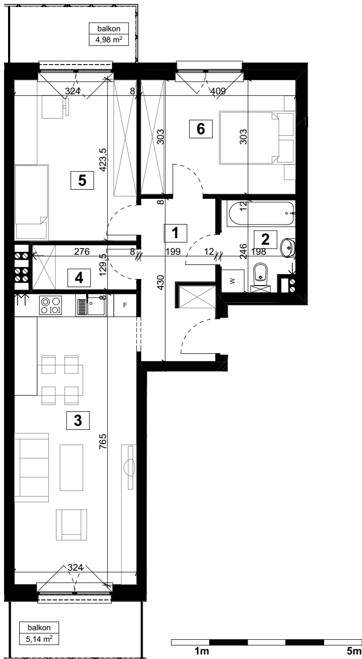
SCHEMAT BUDYNKU
