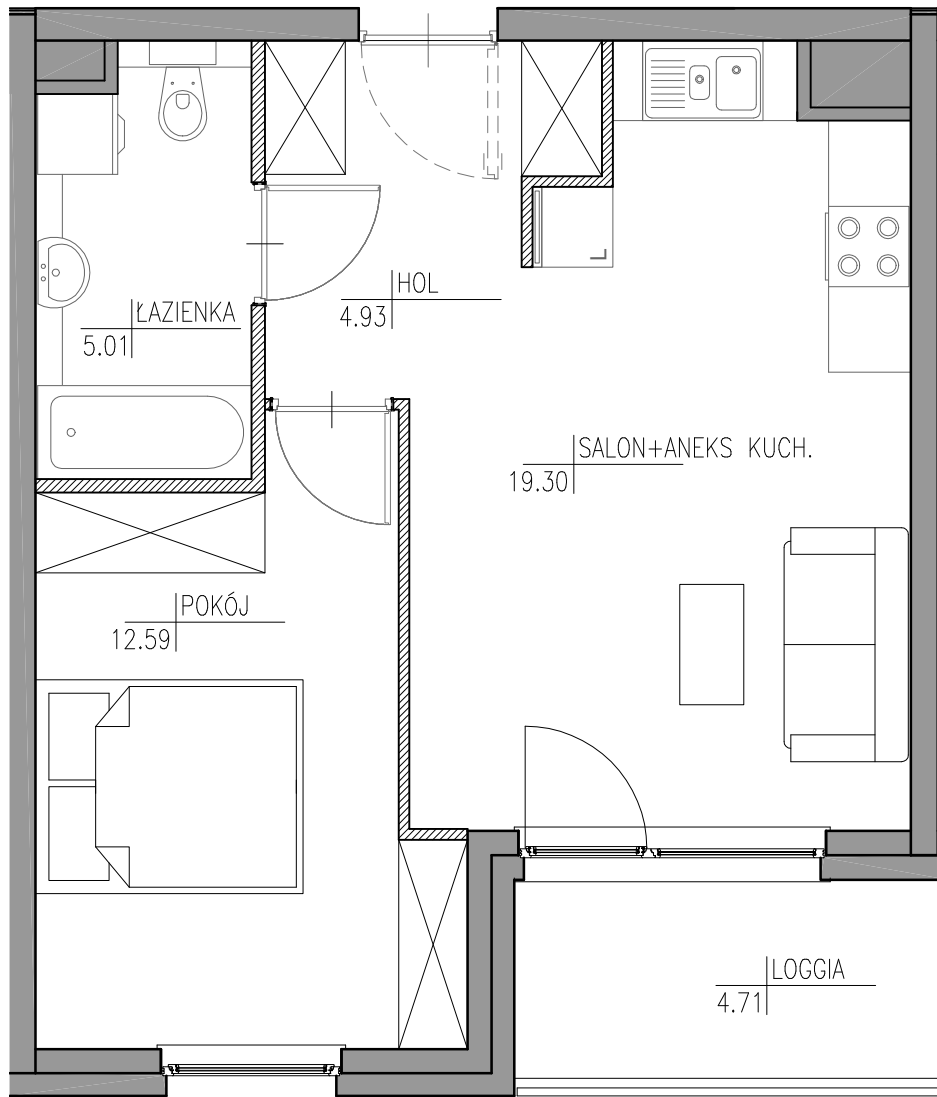
SCHEMAT LOKALU MIESZKALNEGO NA PIĘTRZE
