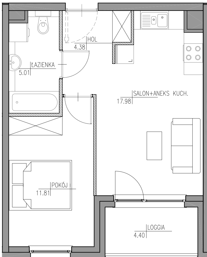
SCHEMAT LOKALU MIESZKALNEGO NA PIĘTRZE
