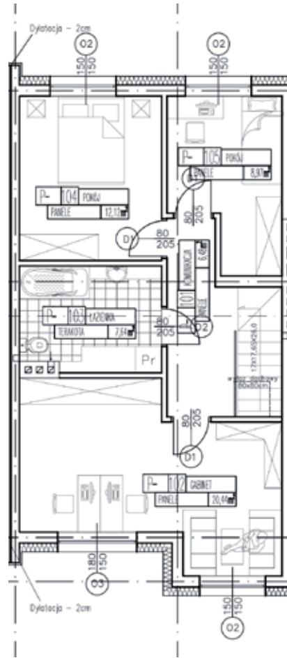
Poddasze
