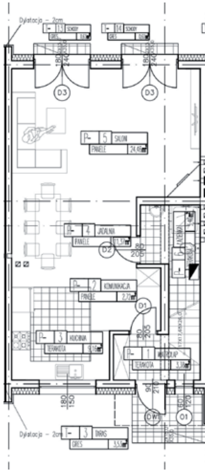
Rzut parteru
