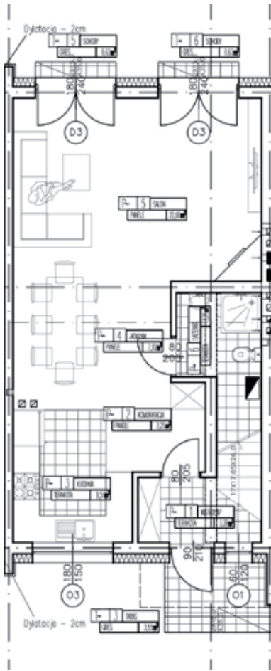
Rzut parteru
