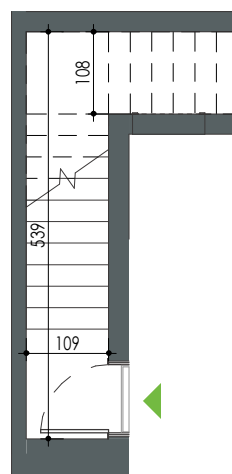
Rzut parteru
