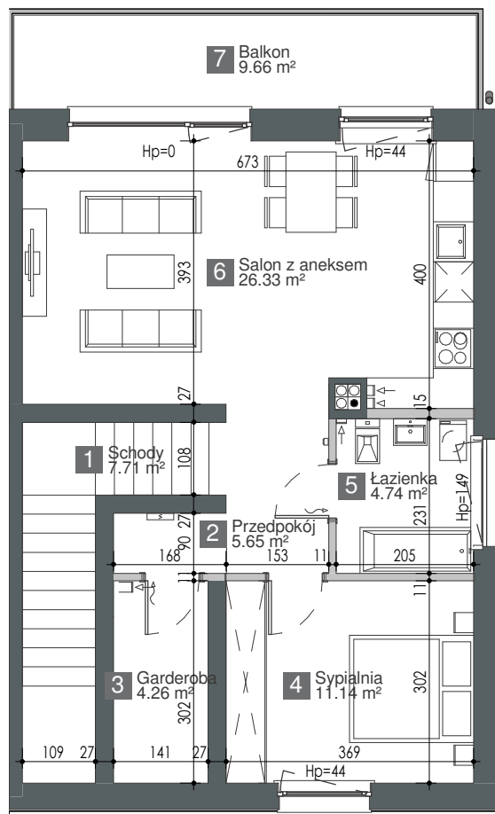
Rzut piętra
